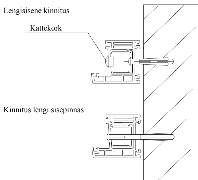
Joonis 5. Kinnitamine läbi akna lengi
